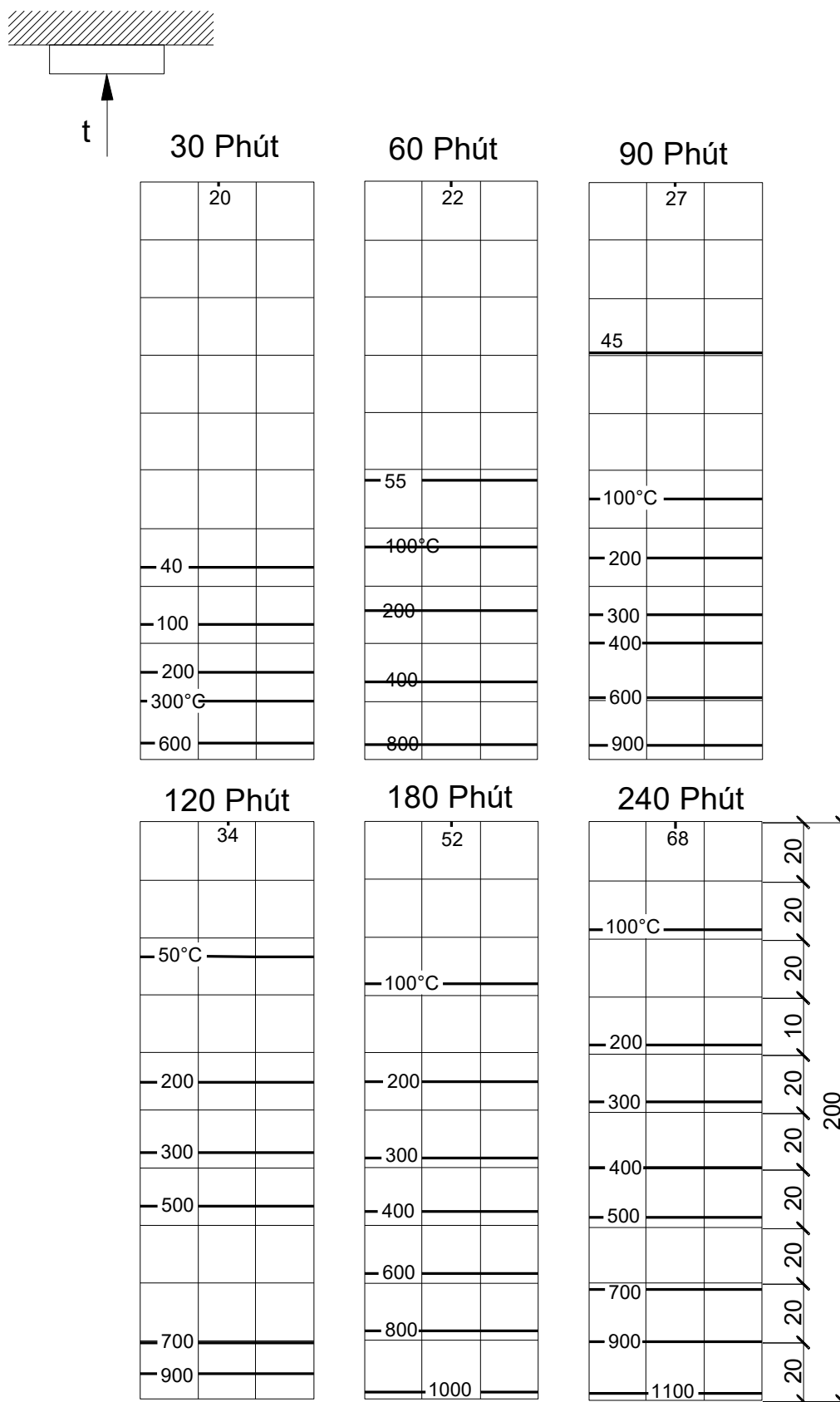
Hình G.12 – Tấm bê tông nặng dày 200 mm khi nung nóng từ một mặt
