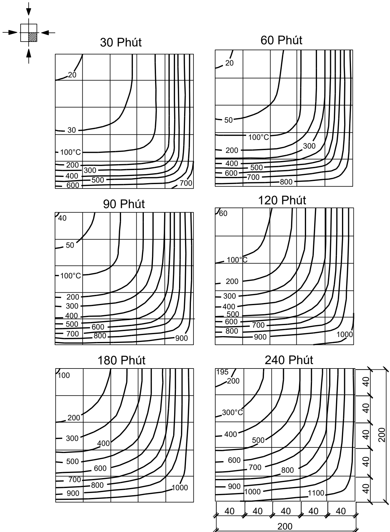
Hình G.2 – Cột bê tông nặng tiết diện 400 mm x 400 mm khi nung nóng từ bốn phía
