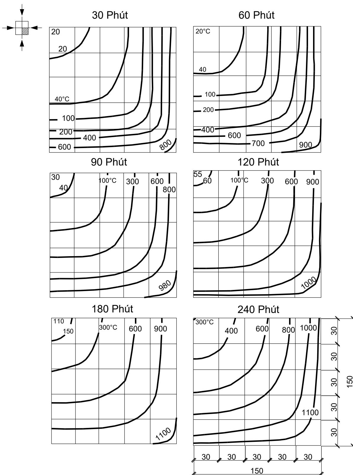
Hình G.3 – Cột bê tông nhẹ tiết diện 300 mm x 300 mm khi nung nóng từ bốn phía
