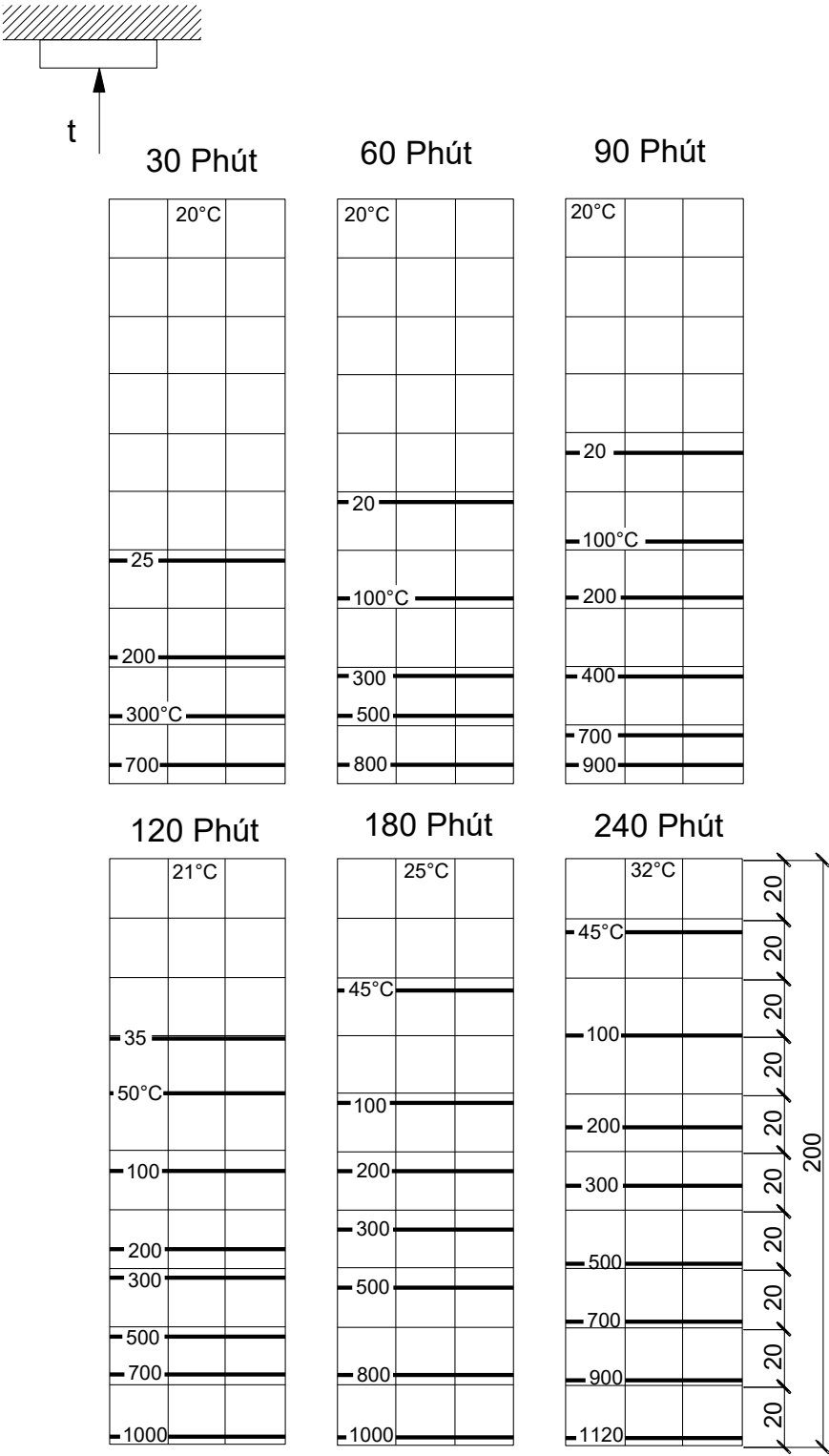
Hình G.15 – Bảng bê tông nhẹ dày 200 mm khi nung nóng với một mặt
