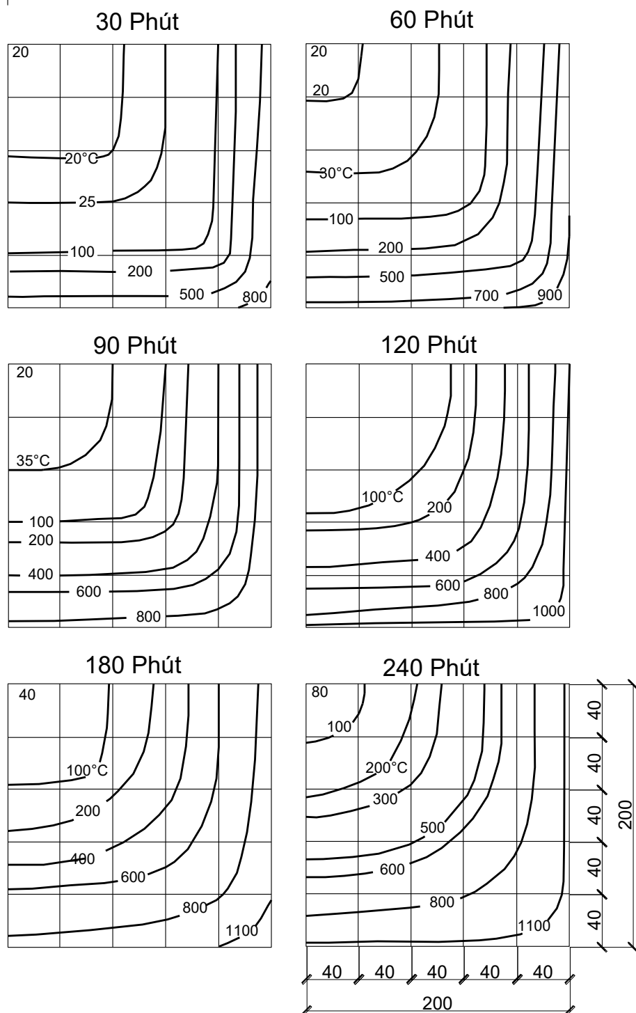
Hình G.9 – Cột bê tông nhẹ tiết diện 400 mm x 400 mm khi nung nóng từ bốn phía
