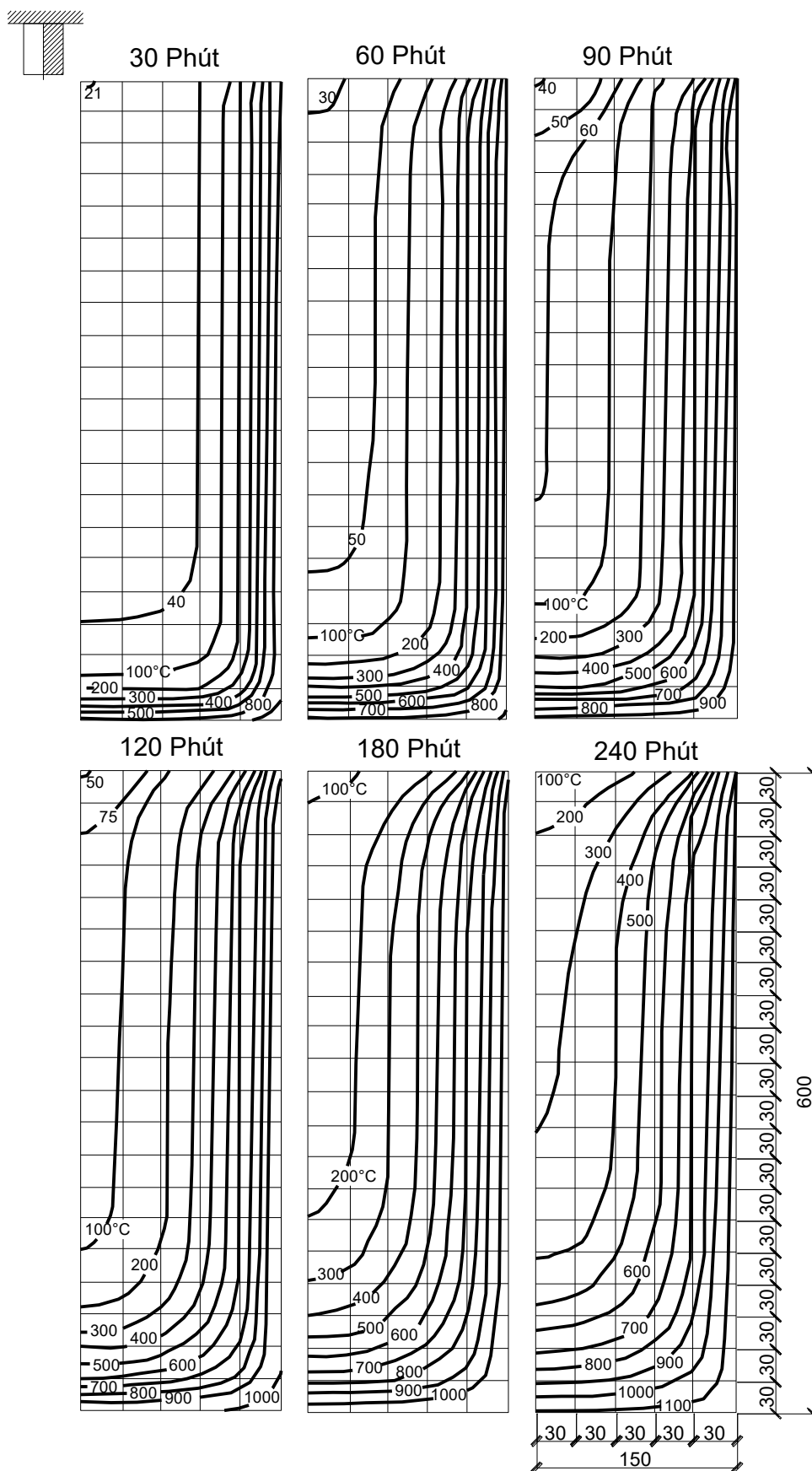
Hình G.7 – Dầm bê tông nặng tiết diện 600x300 mm khi nung nóng từ ba phía
