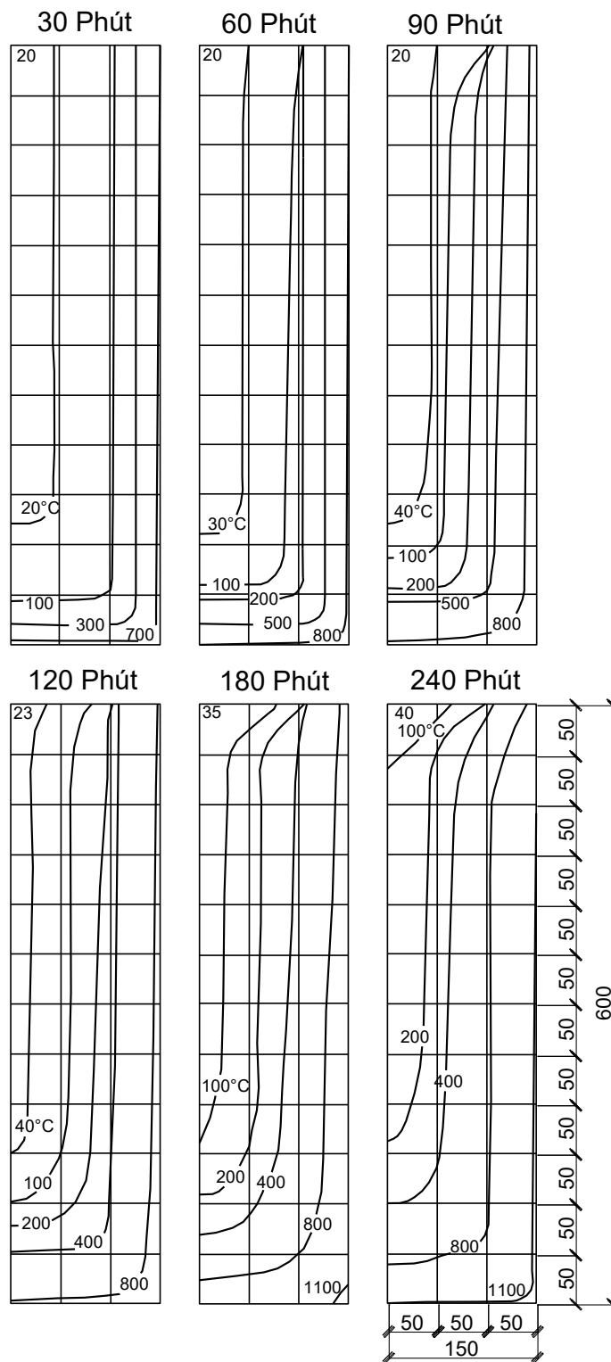
Hình G10 – Dầm bê tông nhẹ tiết diện 600 mm x 300 mm khi nung nóng từ ba phía
