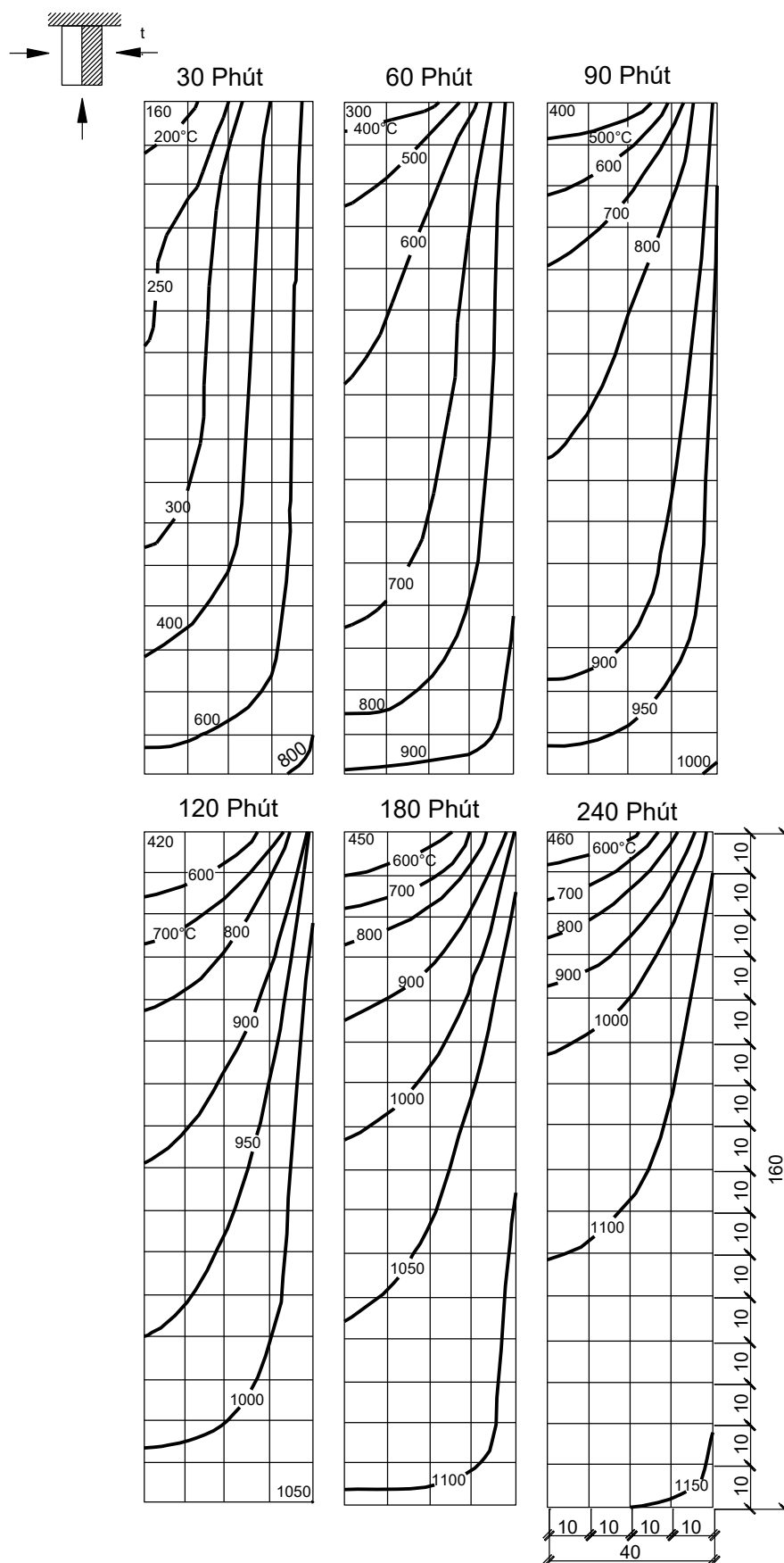
Hình G.5 – Dầm bê tông nặng tiết diện 160 mm x 80 mm khi nung nóng từ ba phía
