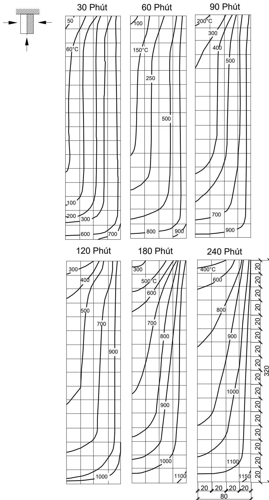
Hình G.6 – Dầm bê tông nặng tiết diện 320 mm x 160 mm khi nung nóng từ ba phía
