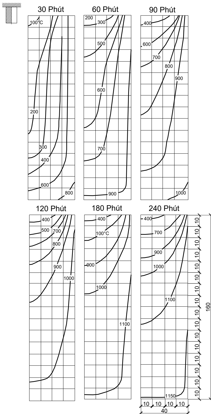
Hình G.8 – Dầm bê tông nhẹ tiết diện 160x80 mm khi nung nóng từ ba phía
