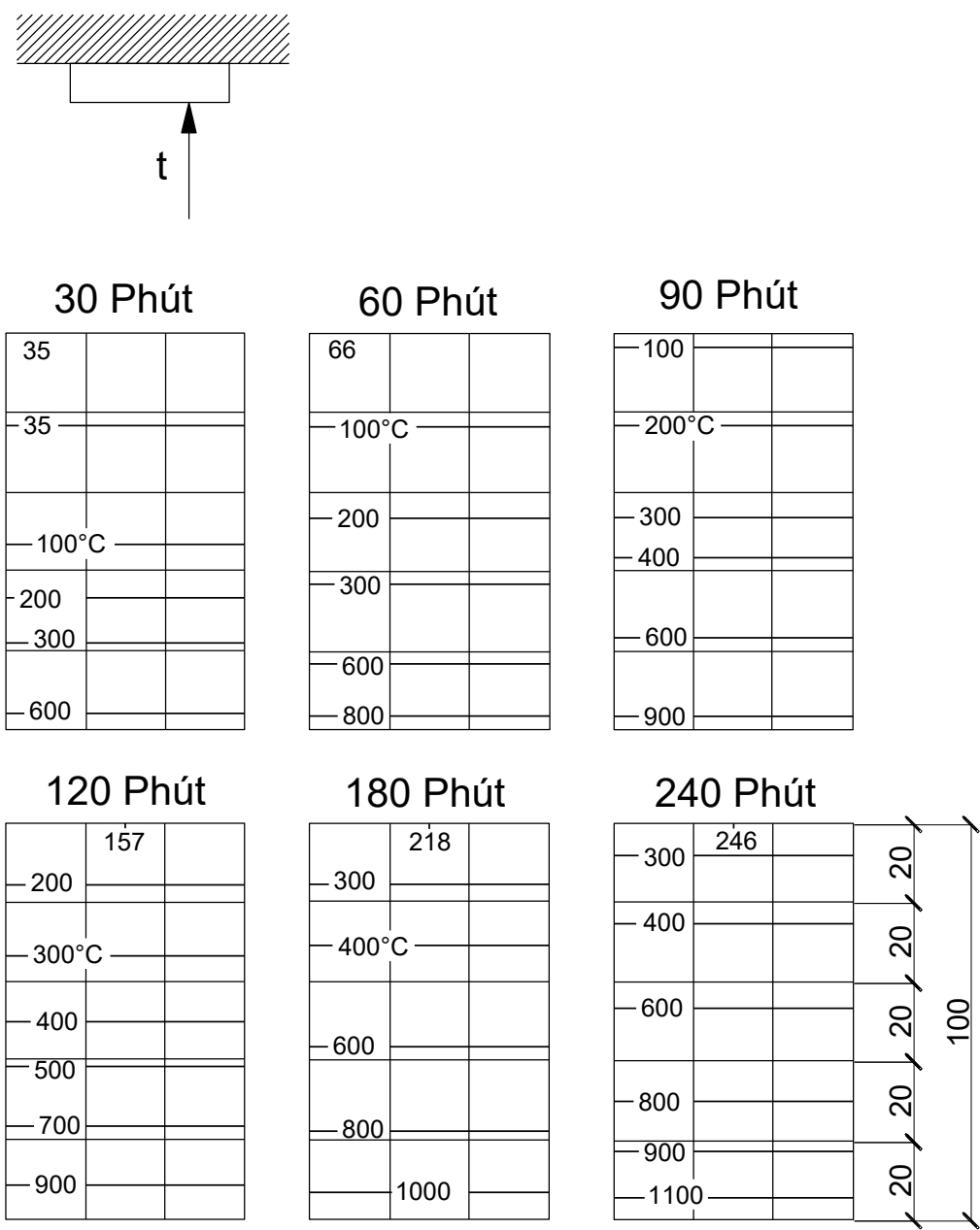
Hình G.11 – Tấm bê tông nặng dày 100 mm khi nung nóng từ một phía
