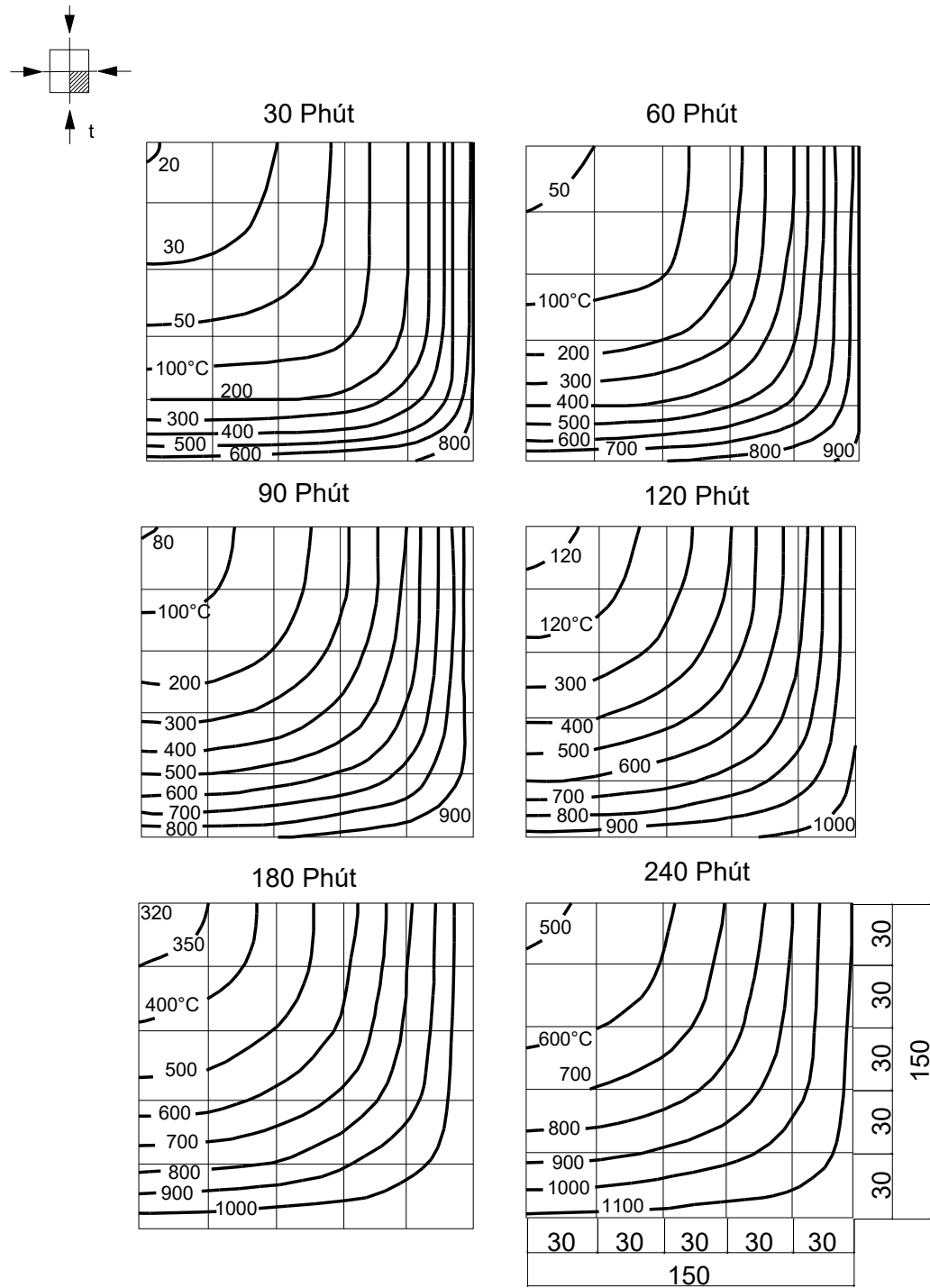
Hình G.1 – Cột bê tông nặng tiết diện 300 mm x 300 mm khi nung nóng từ bốn phía
