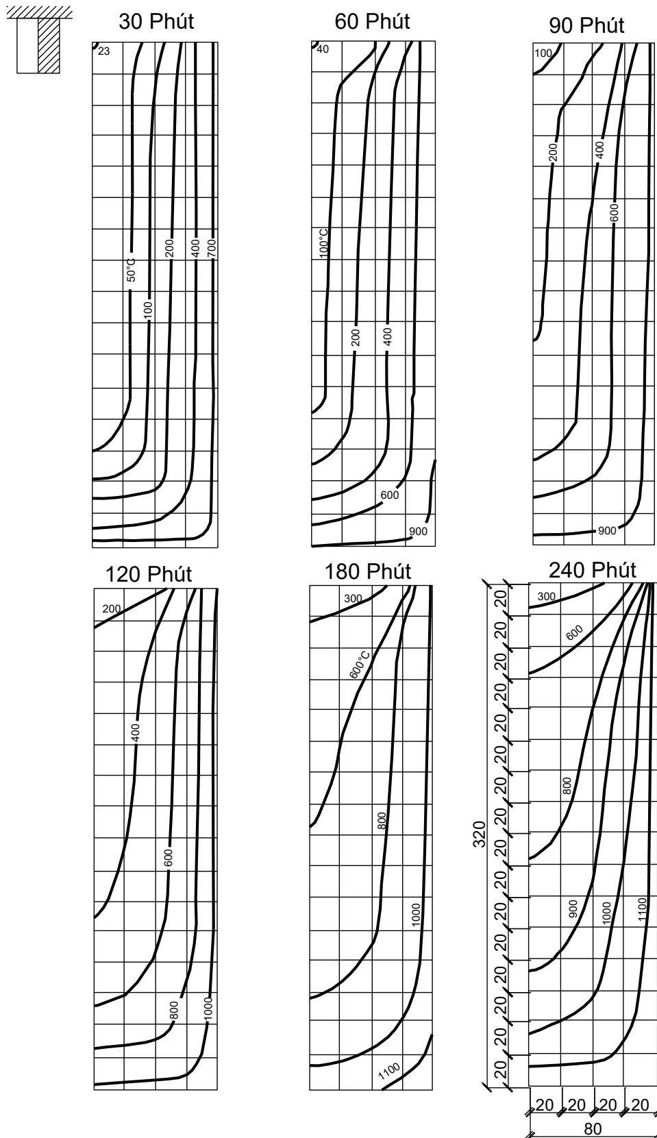
Hình G.4 – Dầm bê tông nhẹ tiết diện 320 mm × 160 mm khi nung nóng từ ba phía
