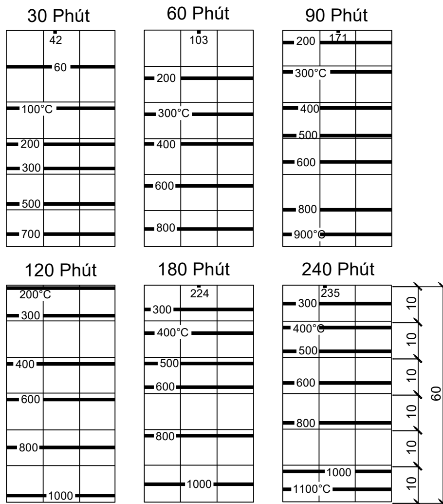
Hình G.13 – Bảng bê tông nhẹ dày 60 mm khi nung nóng với một mặt
