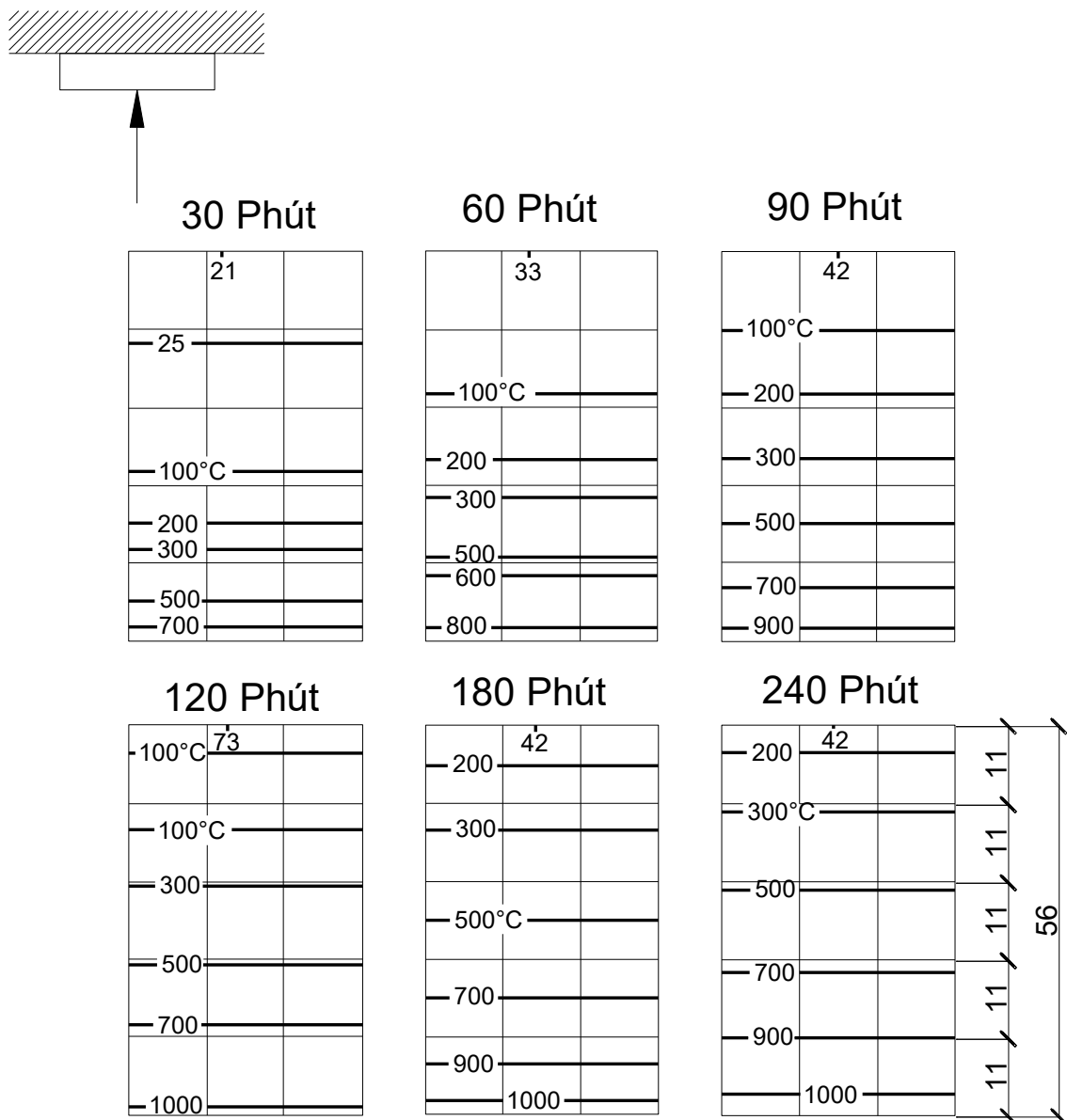
Hình G.14 Bảng bê tông nhẹ dày 100 mm khi nung nóng với một mặt
