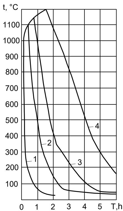
Hình E.5 – Mối quan hệ t - \tau đối với K_l^\tau = 0,08 \text{ m}^{1/2}
