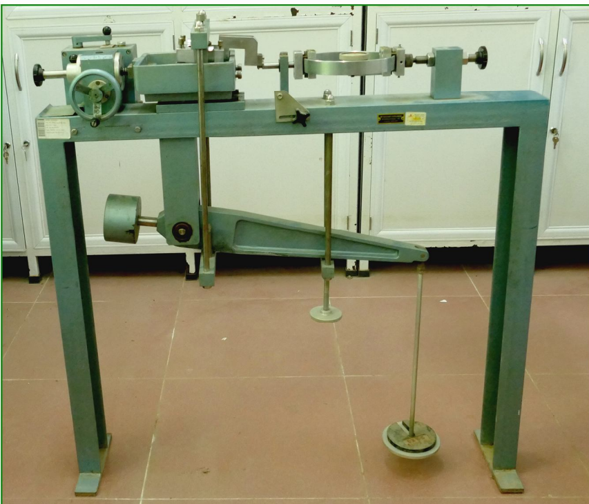
THÍ NGHIỆM CẮT PHẪNG
