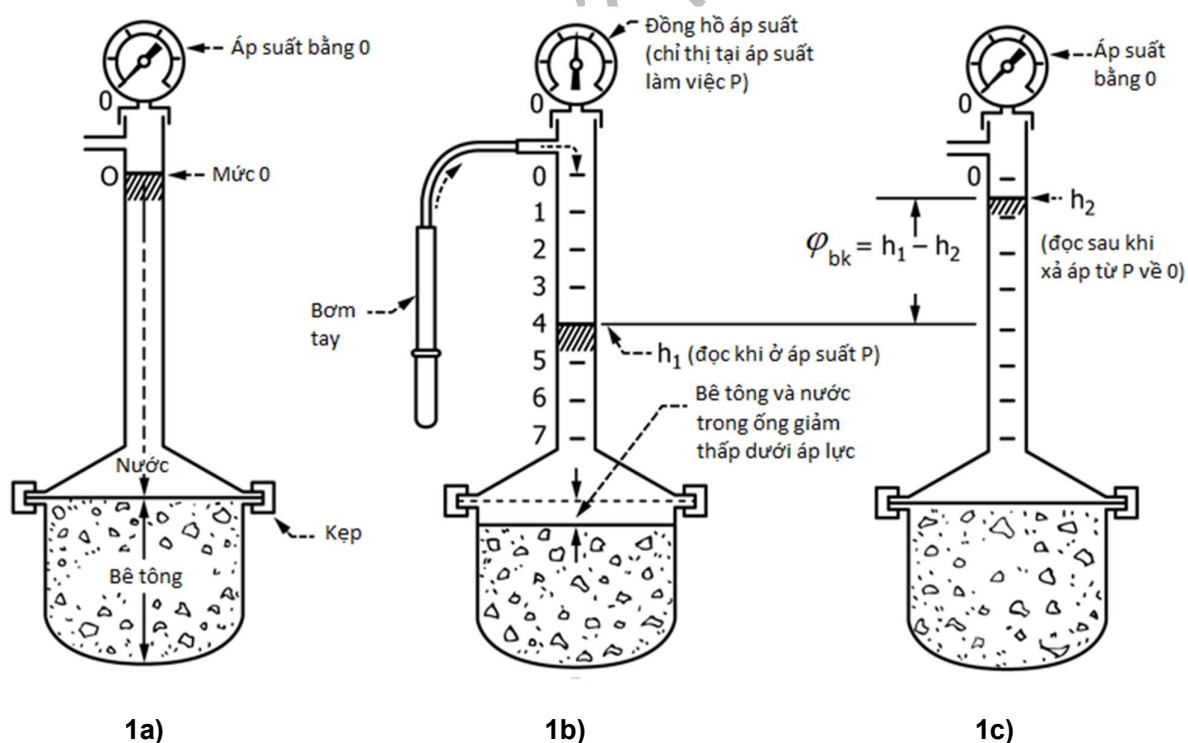
Hình 1 - Sơ đồ bình thử bọt khí kiểu A
