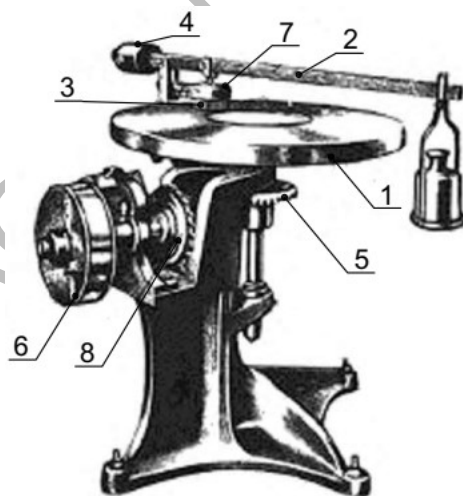
Hình 1 - Sơ đồ máy mài đĩa kiểu LKI-3
