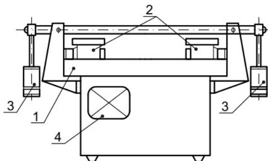
Hình 1 - Sơ đồ máy mài đĩa kiểu LKI-3
