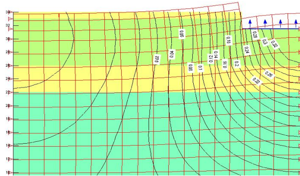
Hình 3. Kết quả tính toán độ lún bằng phần mềm GEOSLOPE
