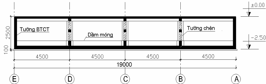
Hình 4. Mặt cắt qua móng
