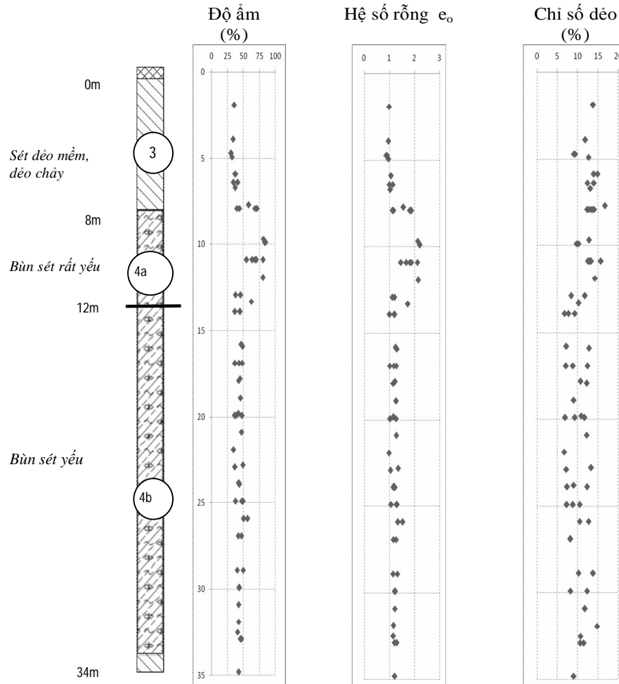
Hình 1. Trụ địa chất điển hình tại khu vực xây dựng
