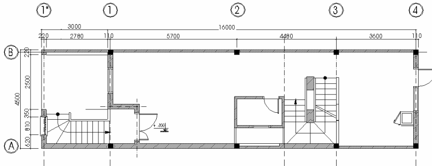
Hình 2. Mặt bằng nhà liền kề
