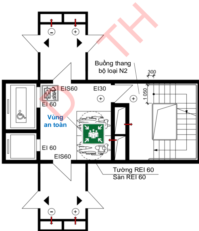
Hình 5 – Bố trí vùng an toàn trong sảnh thang máy chữa cháy bên cạnh là buồng thang bộ loại N2 [8]
