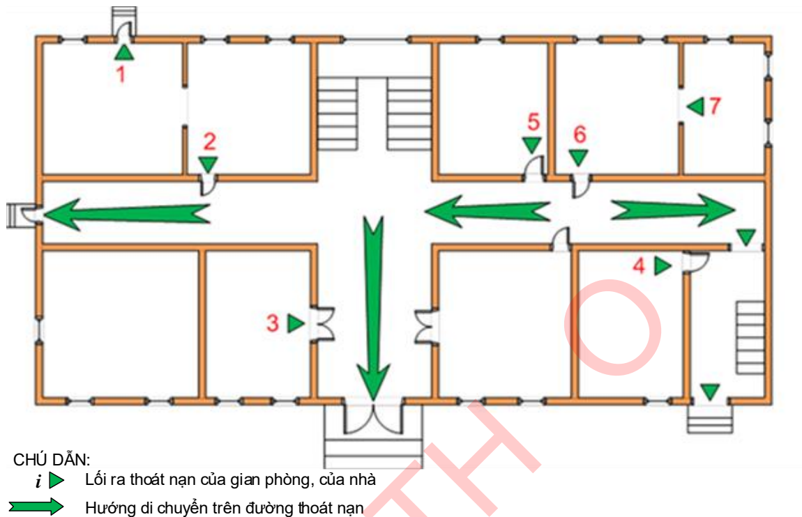
Hình 23 – Ví dụ minh họa về các lối ra thoát nạn của gian phòng và của nhà tại tầng có lối ra bên ngoài (tầng 1)
