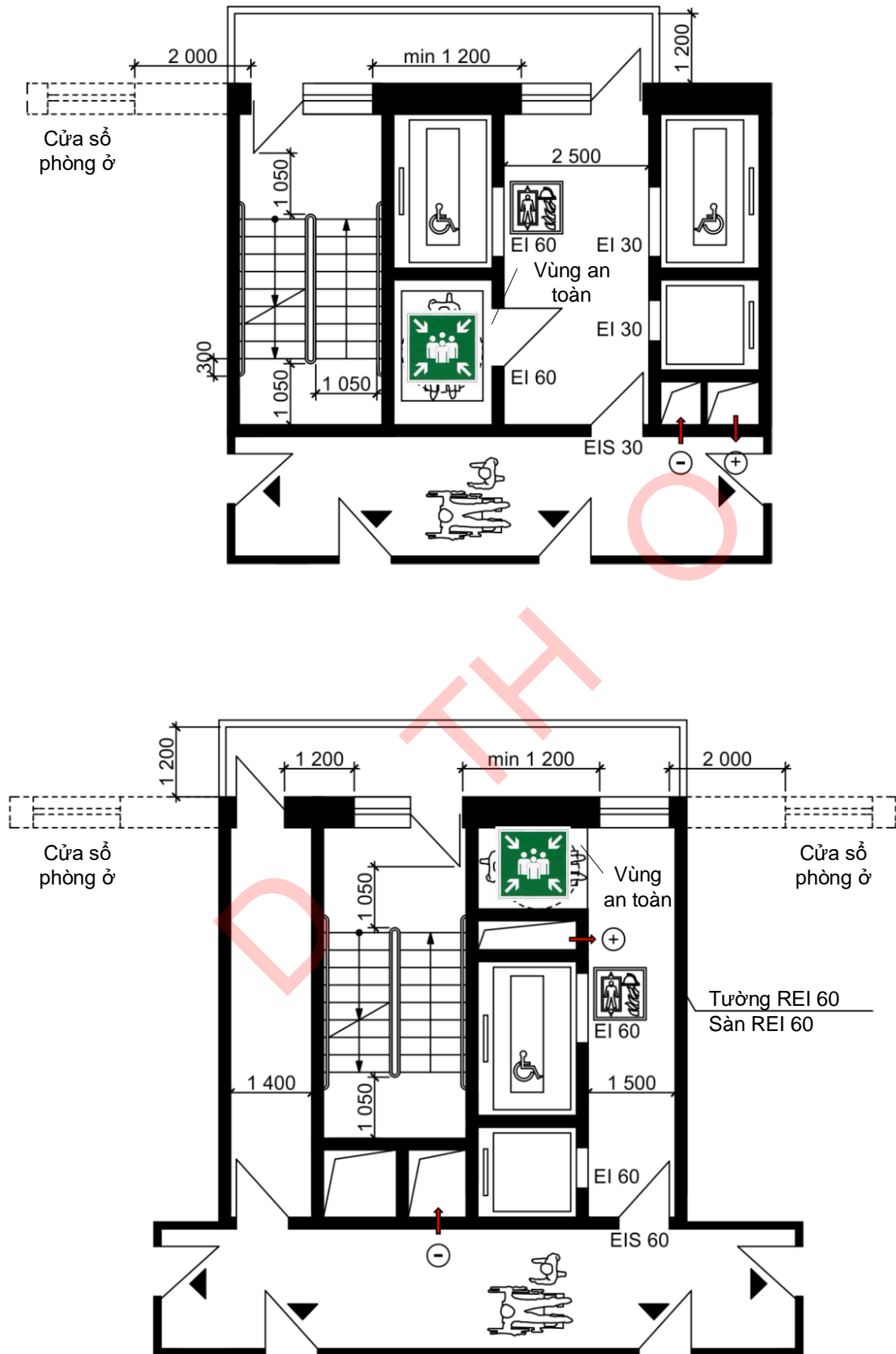
Hình 4 – Bố trí vùng an toàn trong sảnh thang máy chữa cháy bên cạnh buồng thang bộ loại N1 [8]
