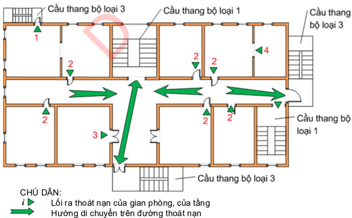
Hình 24 – Ví dụ minh họa về lối ra thoát nạn của gian phòng và của tầng khác với tầng có lối thoát bên ngoài (tầng 1)
