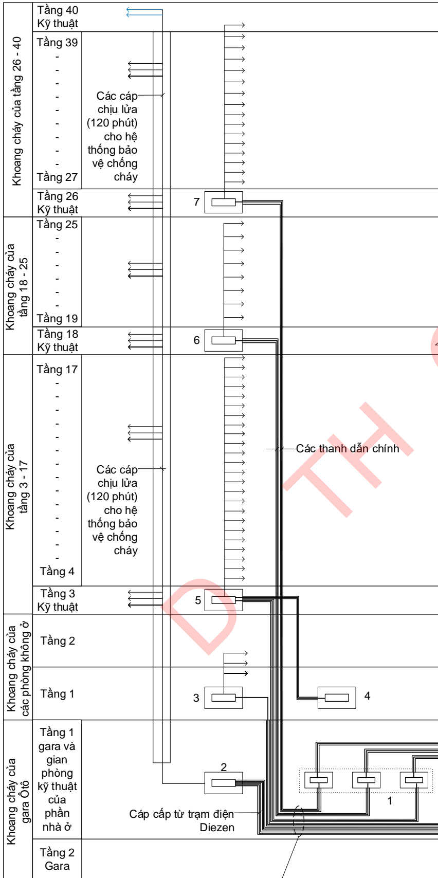
Hình 57 – Sơ đồ nguyên lý (cấu trúc) đặt mạng lưới điện 380/220 V (mặt cắt đứng) cho nhà cao tầng [29]
