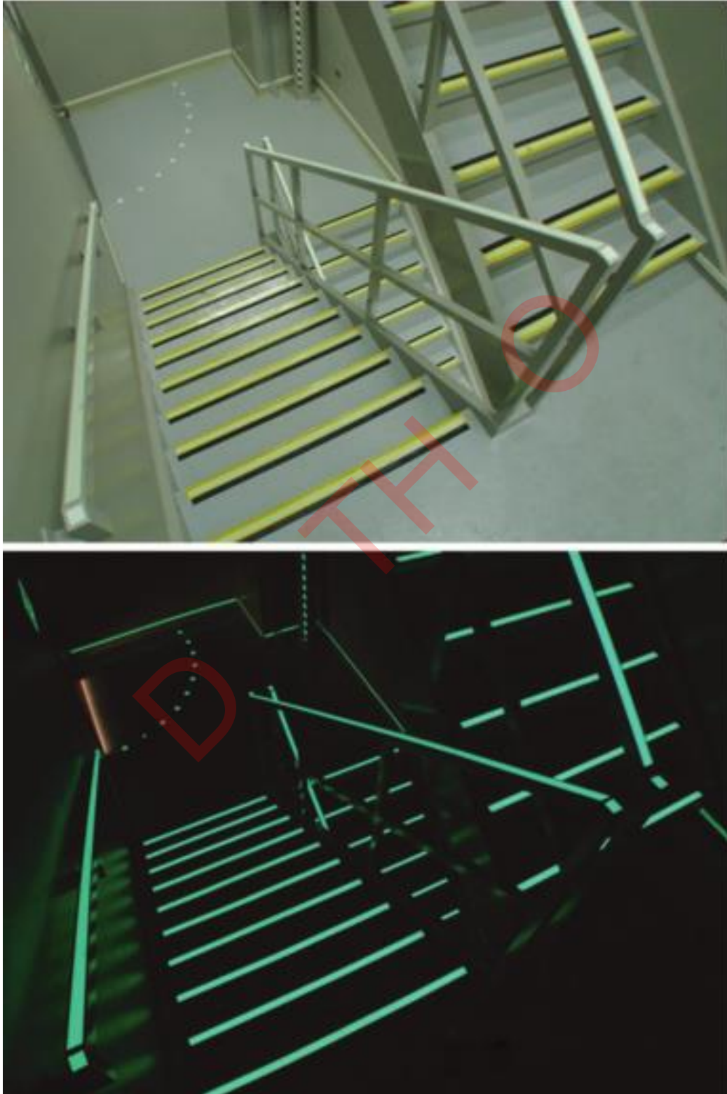
Hình 58 – Ví dụ về đánh dấu các chi tiết cầu thang bộ thoát nạn bằng vật liệu phát sáng [39]
