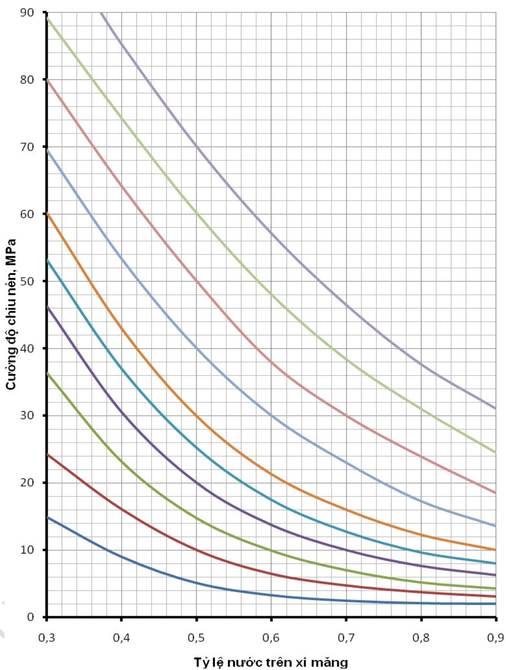
Hình 2 - Lựa chọn tỷ lệ nước trên xi măng
