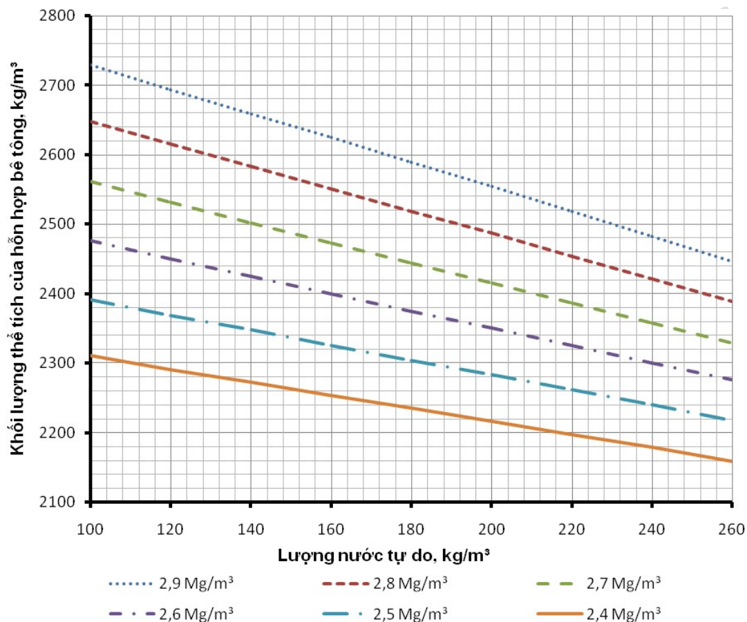
Hình 6 - Lựa chọn khối lượng thể tích của hỗn hợp bê tông
