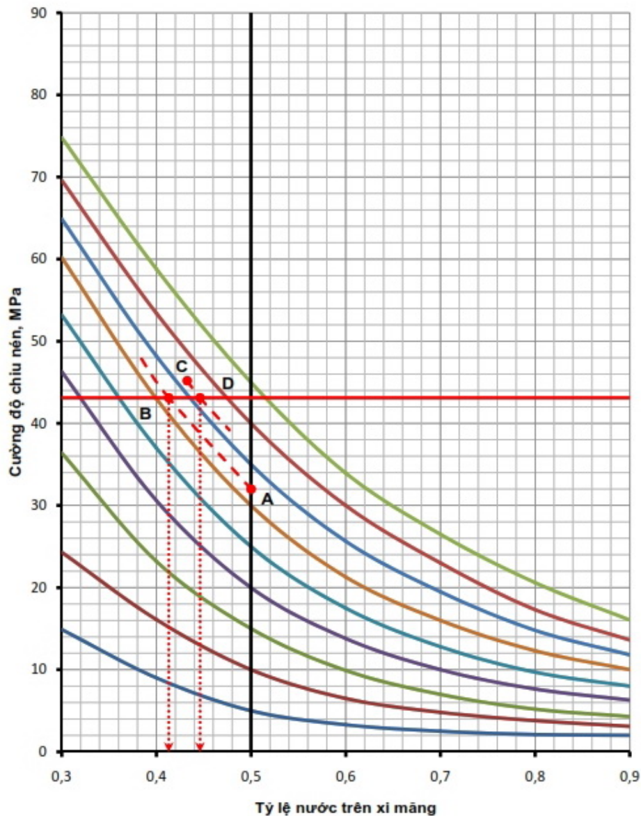
Hình A.1 - Lựa chọn tỷ lệ nước trên xi măng
