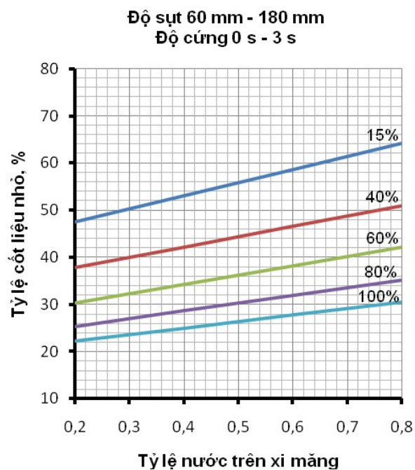
Hình 4 - Tỷ lệ cốt liệu nhỏ khi kích thước hạt lớn nhất của cốt liệu lớn bằng 20 mm
