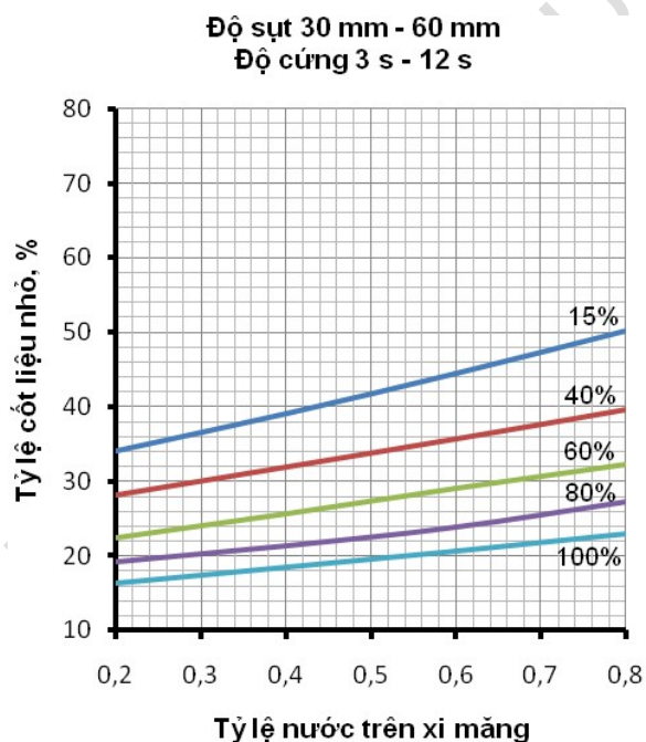
Hình 5 - Tỷ lệ cốt liệu nhỏ khi kích thước hạt lớn nhất của cốt liệu lớn bằng 40 mm
