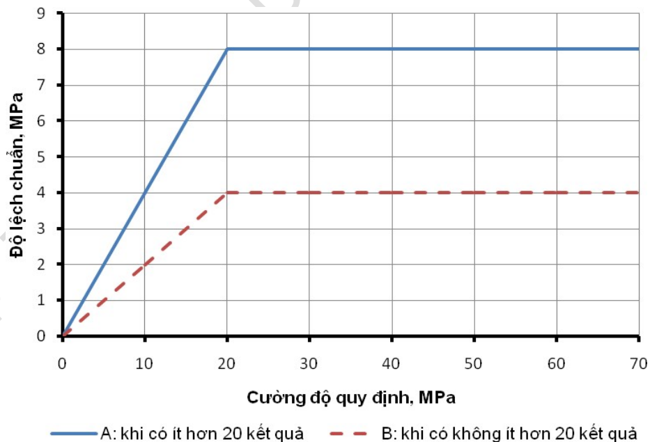
Hình 1 - Tương quan giữa độ lệch chuẩn và cường độ quy định
