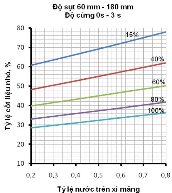
Hình 3 - Tỷ lệ cốt liệu nhỏ khi kích thước hạt lớn nhất của cốt liệu lớn bằng 10 mm
