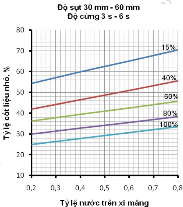
Hình 3 - Tỷ lệ cốt liệu nhỏ khi kích thước hạt lớn nhất của cốt liệu lớn bằng 10 mm
