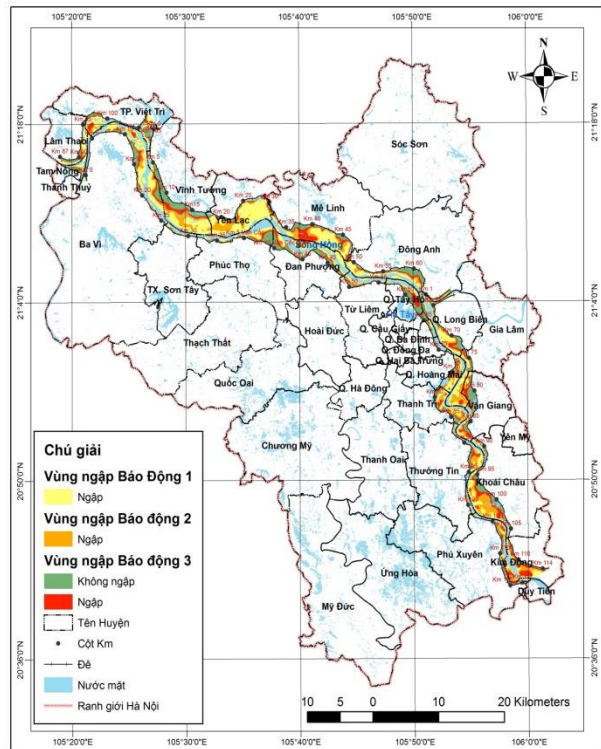
Hình 15. Bản đồ phân vùng ngập lụt
