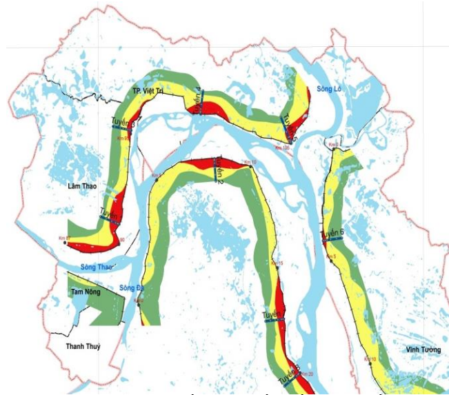
Hình 7. Vị trí tuyến quan trắc biến dạng thắm
