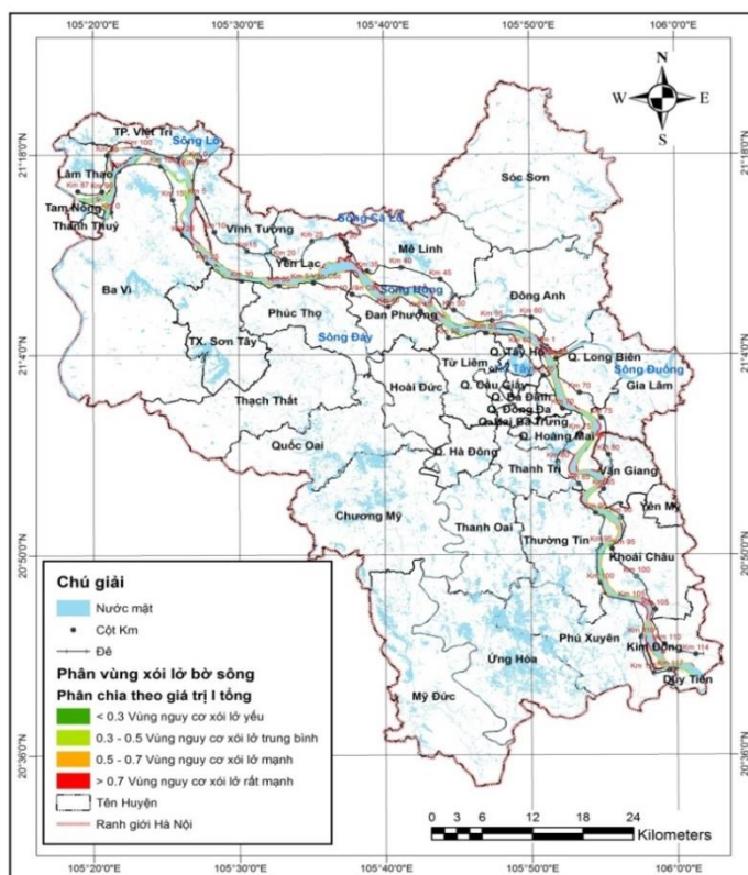
Hình 12. Bản đồ phân vùng xói lở theo giá trị ( I_5 )
