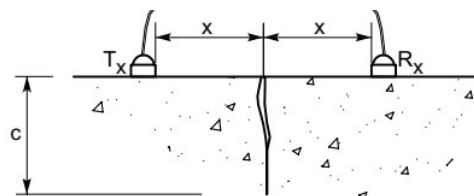
b) Bố trí đầu dò ước tính chiều sâu vết nứt
