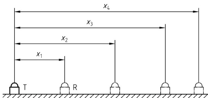
a) Bố trí đầu dò xác định chiều dày lớp bê tông bề mặt chất lượng kém
