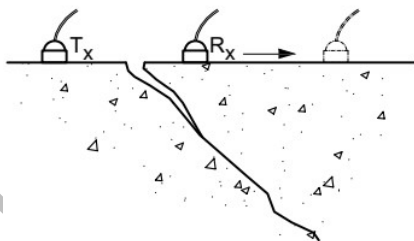
a) Bố trí đầu dò xác định vết nứt xiên
