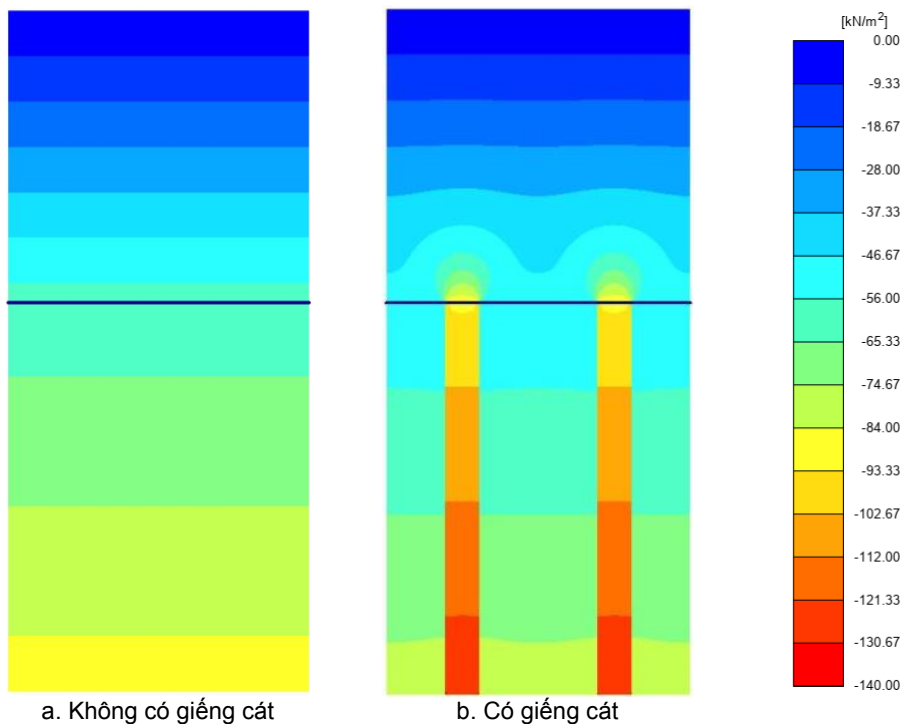
Hình 4. Ứng suất hữu hiệu theo phương thẳng đứng \sigma'_z ( \text{kN/m}^2 )
