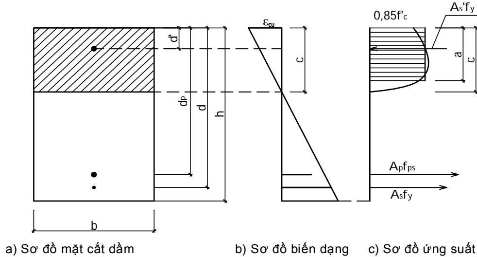
Hình 2. Sơ đồ tính toán tiết diện dầm tại trạng thái chịu uốn cực hạn
